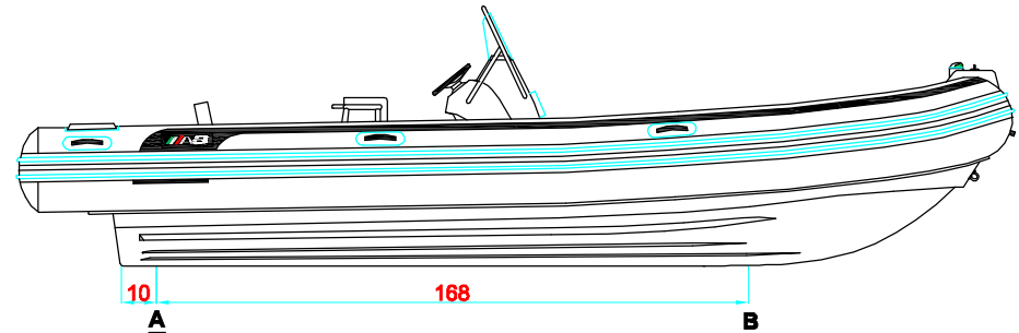
LONGITUDINAL PROFILE PERFIL LONGITUDINAL
